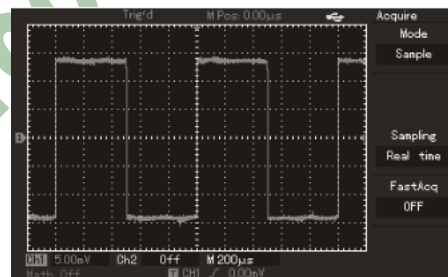
Figura 3-4 Reducción de ruido random de la señal
