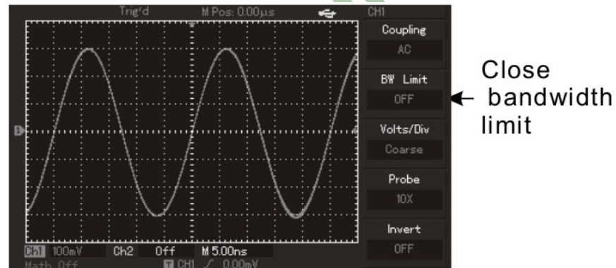
Figura 2-4 Forma de onda con ancho de banda máximo
