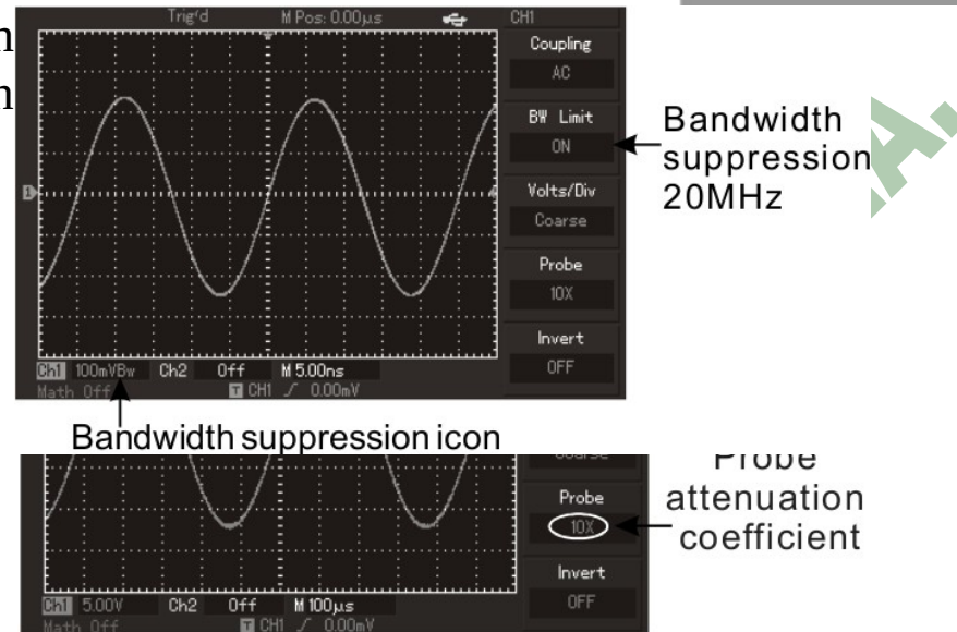
Figura 2-5 Forma de onda con ancho de banda limitado a 20MHz
