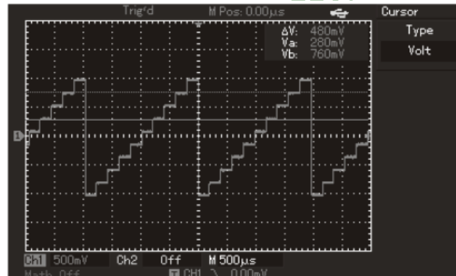
Figura 3-6 Medición de diferencia de tensiones con el cursor
