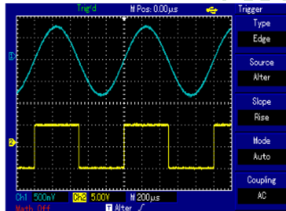
Figura 2 - 16 Observación de dos señales de diferente frecuencia mediante disparo alternado
