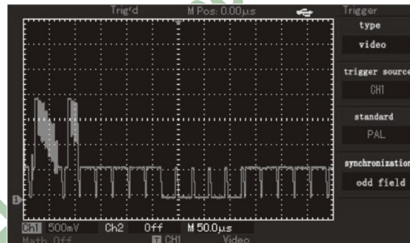
Figura 3-8 Disparo de campo o vertical
