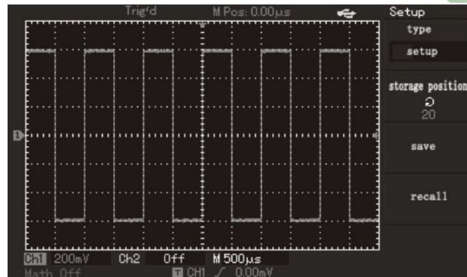
Figura 3-10 Configuración de la función almacenamiento
