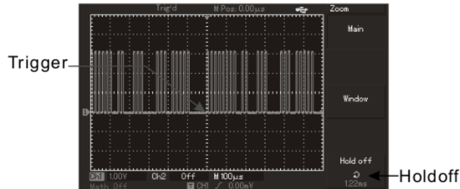
Figura 2—17 Hold off usado para sincronizar formas de onda complejas
