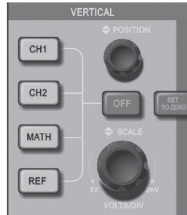
Figura 3-13 Control del vertical para equipos con display de 5,7”
