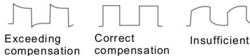
Figura 1 – 8 Corrección de Compensación de la punta de pruebas
