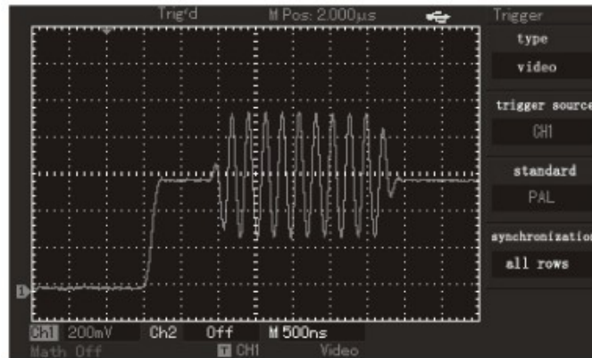
Figura 2-14 Disparo de video: sincronización de fila
