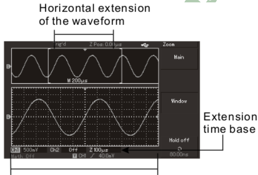
Figura 2 - 12 Display con ventana extendida
