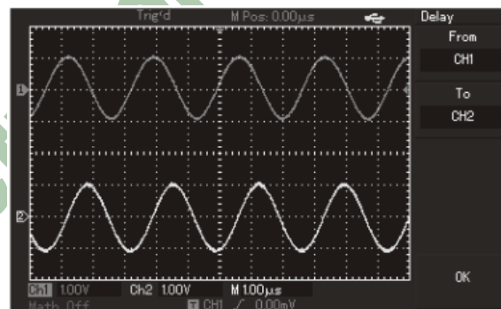
Figura 3-2: Delay causado por el circuito
