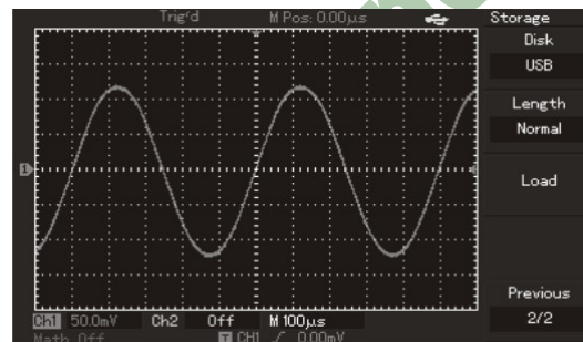
Figura 3-12 Almacenamiento de señales en disco USB
