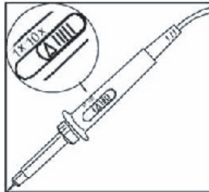
Figura 1 - 5 Configuración de la atenuación de la punta de pruebas
