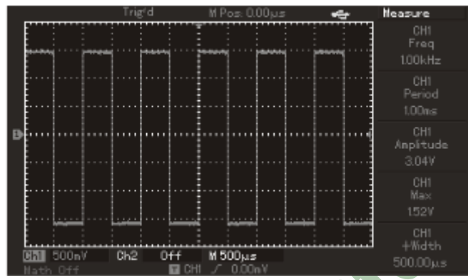
Figura 3-15 Copia de pantalla
