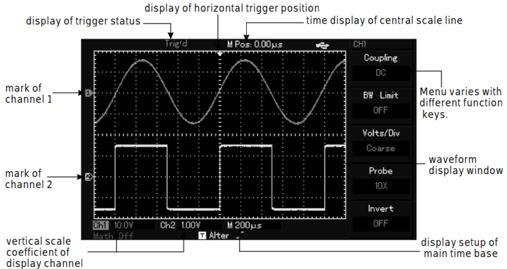
Diagrama de la interfaz de display de los osciloscopios digitales (UTD2000L)
