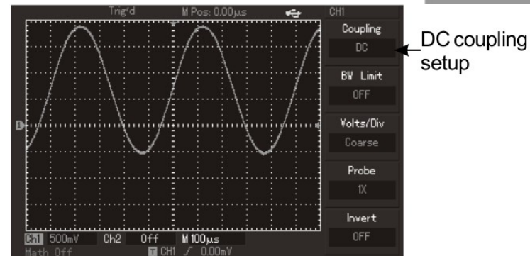
Figura 2- 2 Señal senoidal con componente DC
