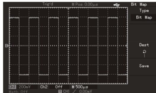
Figura 3-11 Almacenamiento de señales
