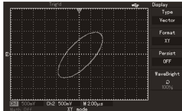
Figura 2 -13 Display en modo X-Y
