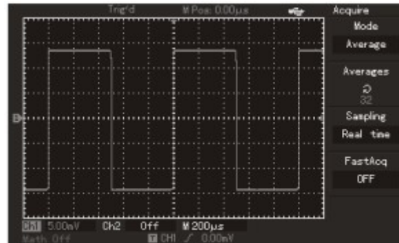
Figura 3-5 Reducción de ruido de la señal
