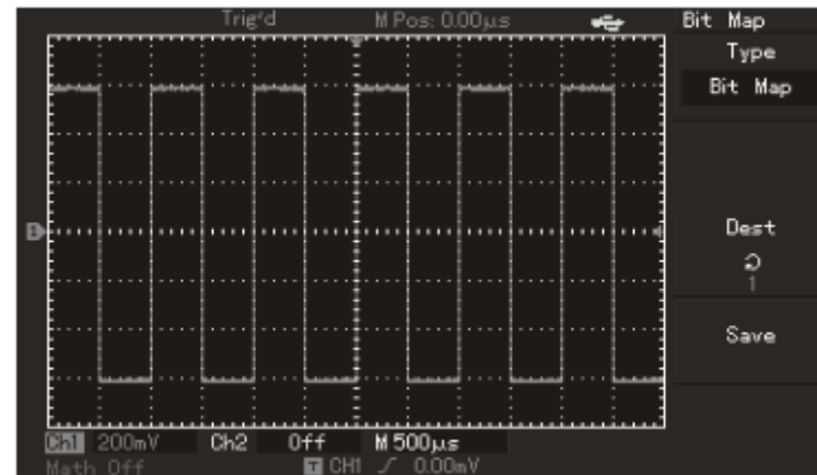
Figura 2-25 Configuración de almacenamiento
